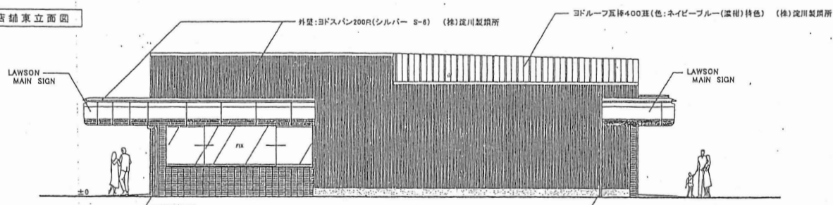
店舗北立面図
